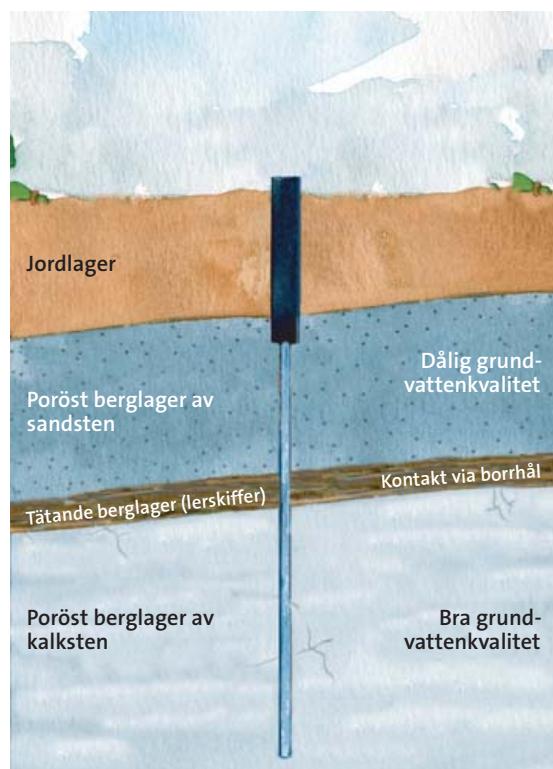
Figur 4. Olika sedimentära bergarter är ofta lagrade på varandra. Skiffer kan utgöra täta skikt mellan vattenförande lager så att vatten av god kvalitet inte blandas med sämre vatten.
